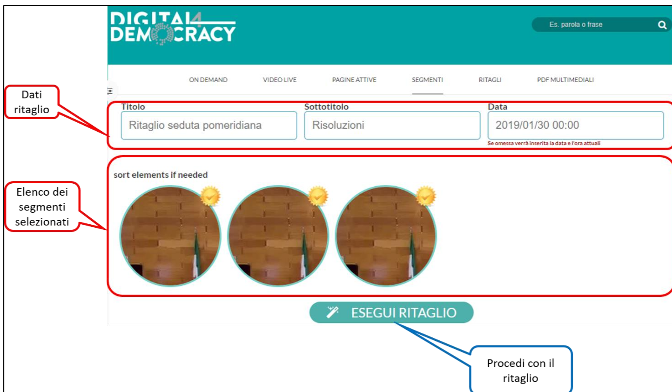
Figura 22 - Esegui ritaglio
