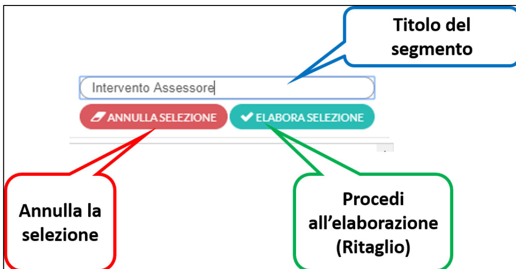
Figura 19 - Elaborazione Selezione
