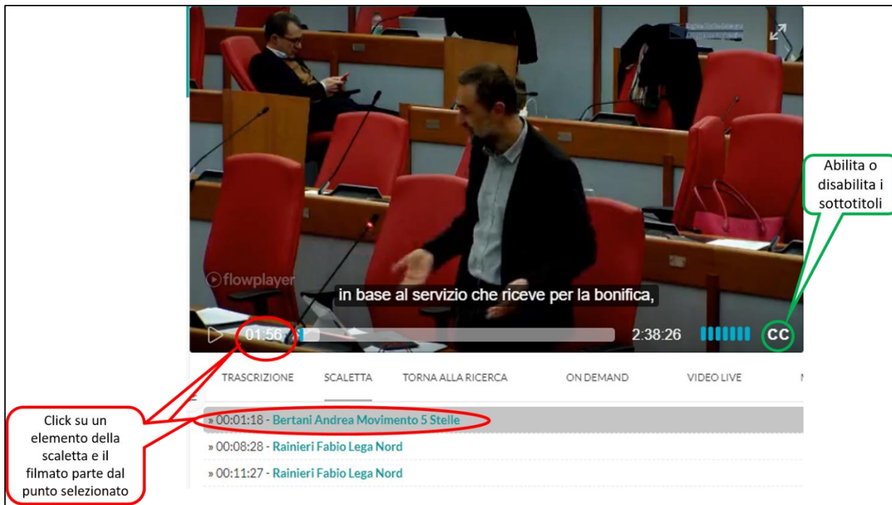
Figura 15 - Scaletta
