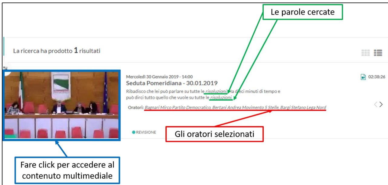
Figura 7 - Risultato ricerca
