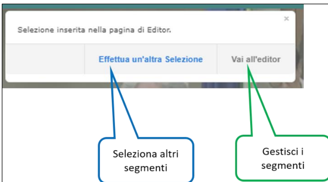
Figura 20 - Segmento Elaborato
