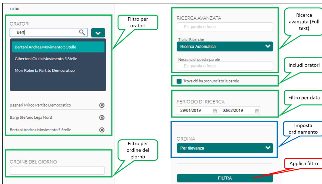
Figura 5 - Opzioni Ricerca
