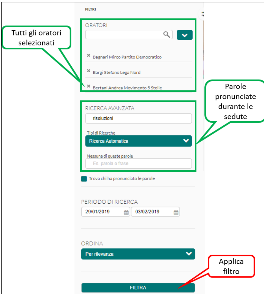
Figura 6 - Esempio ricerca
