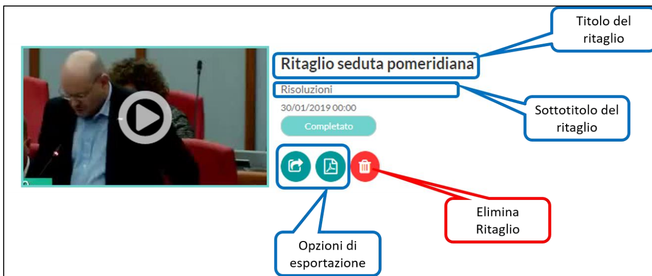
Figura 24 - Ritaglio completato
