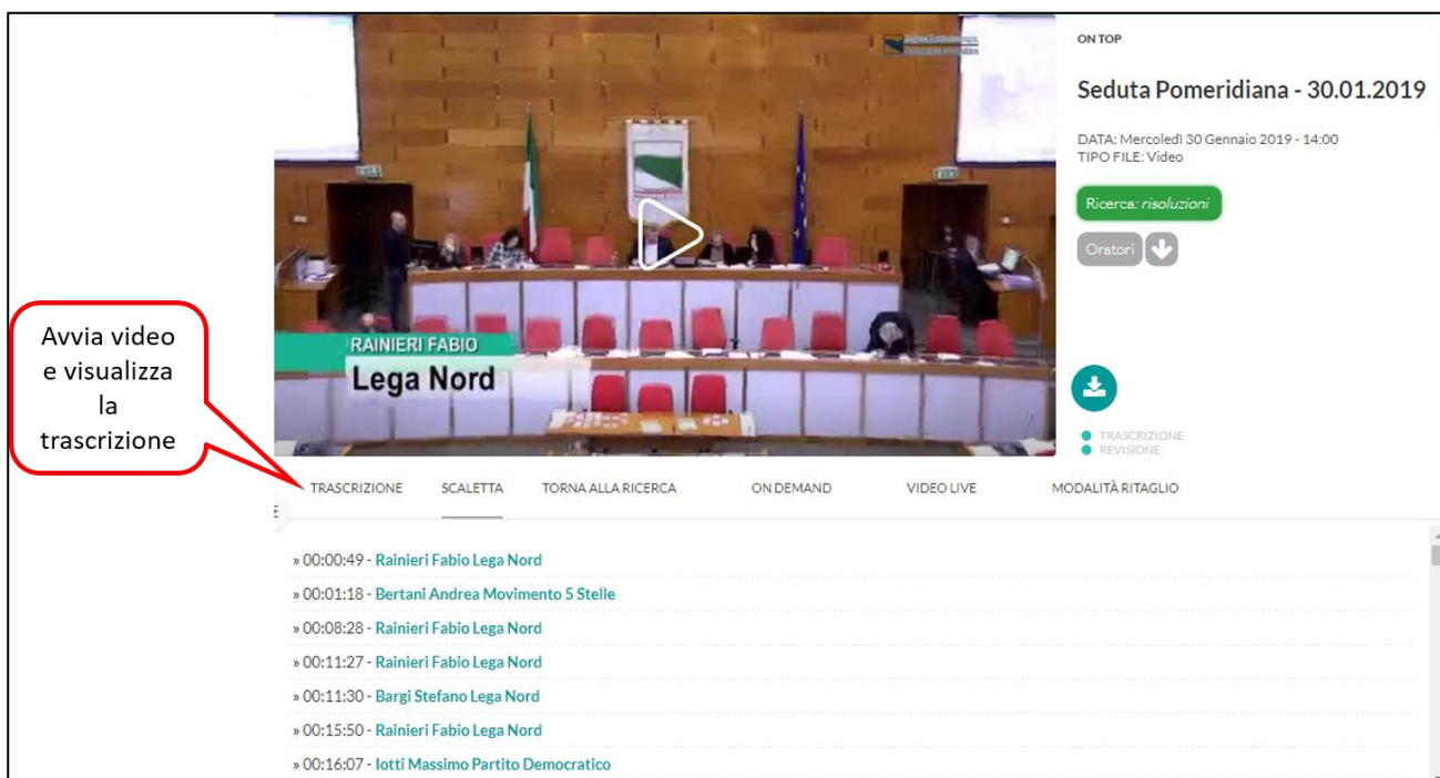
Figura 8 – Dettaglio
