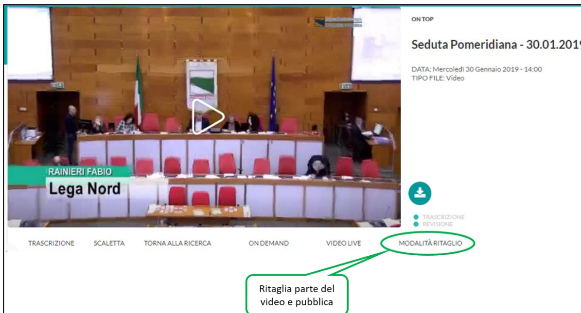
Figura 16 - Funzionalità avanzate
